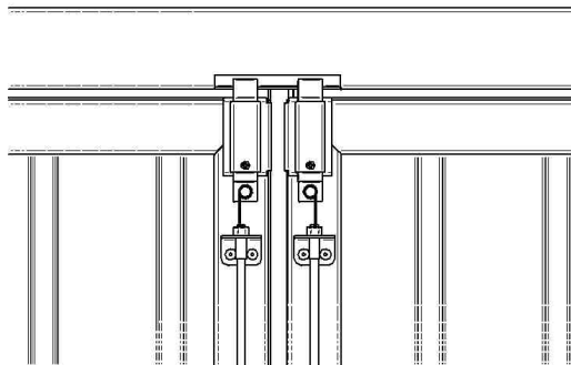
Rys.4 Ustawienie równej odległości pomiędzy skrzydłami bramy a ościeżnicą.
