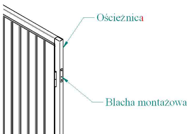
Rys.1 Blacha montażowa
