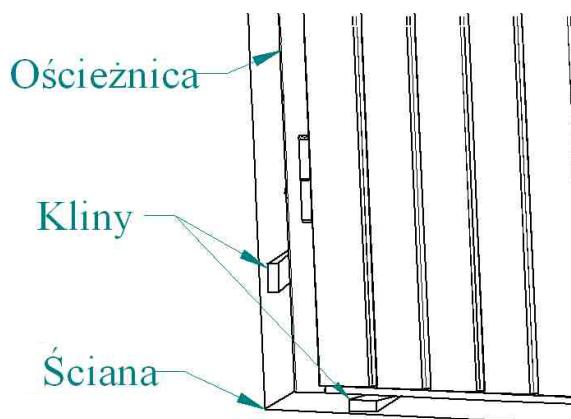
Rys.3 Ustawianie drzwi w otworze za pomocą klinów
