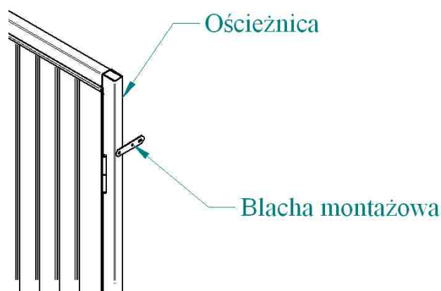
Rys.2 Blacha montażowa ustawiona
