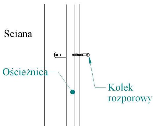
Rys.5 Mocowanie ościeżnicy bramy do ściany.
